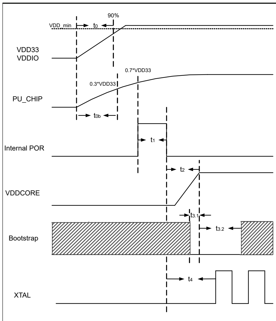
图 6.2: 上电时序 2
