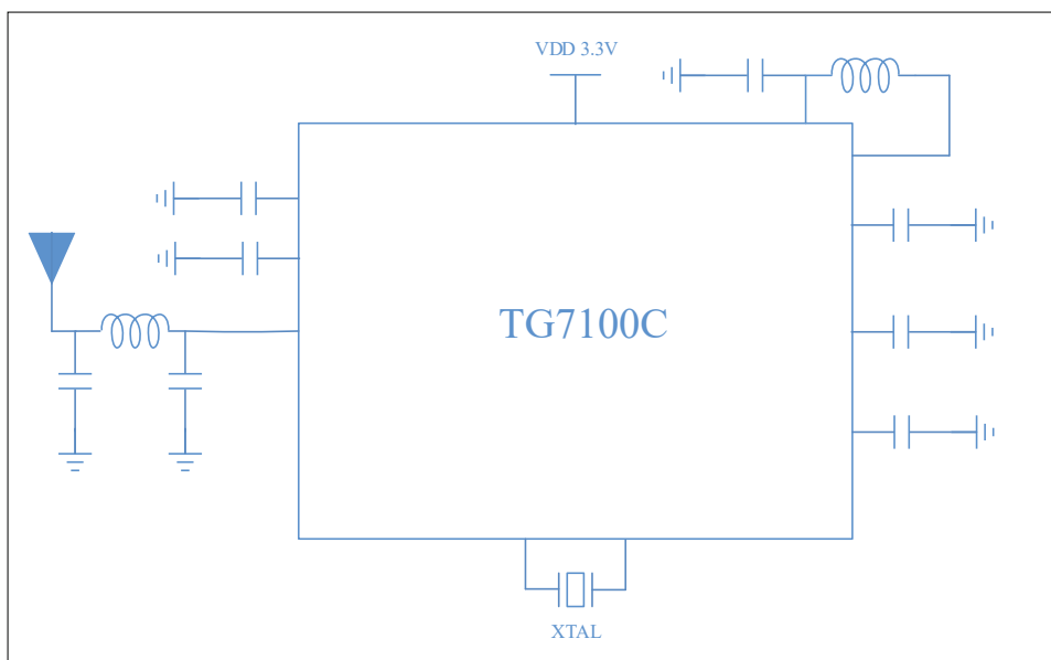
图 8.1: 参考设计
