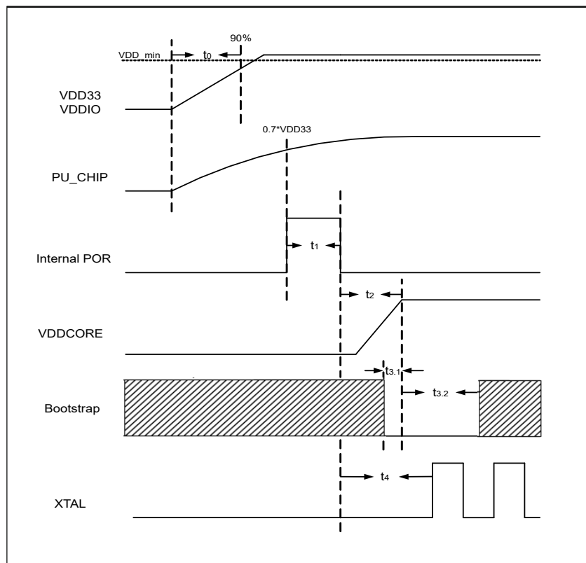
图 6.1: 上电时序 1
