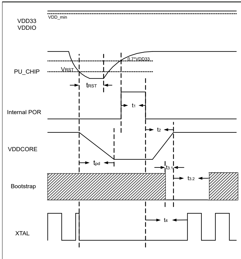
图 6.3: 复位时序
